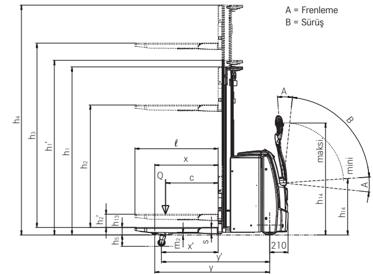
Yan görünüş
